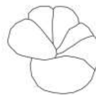
Cibicides lobatulus
