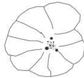
Cribrostomoides crassimargo
