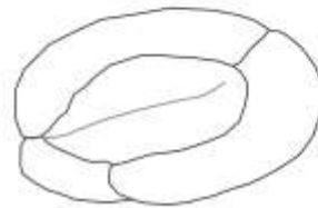
Qunqueloculina seminulum
